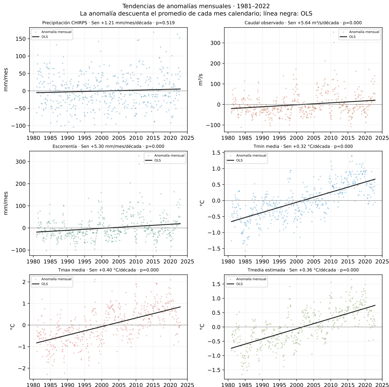
Figura 16: Anomalías mensuales y recta OLS, 1981–2022. Los títulos presentan la pendiente de Sen estacional por década y el valor p de Mann–Kendall estacional.
