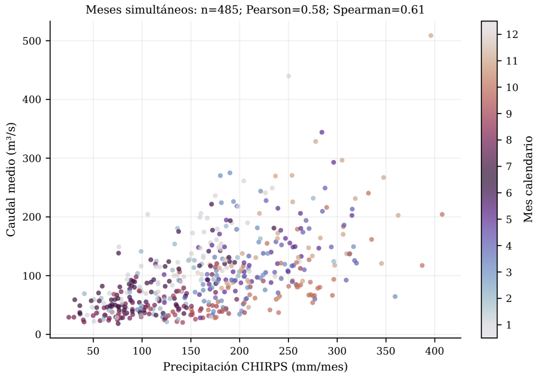
Figura 15: Dispersión de P CHIRPS y Q observado. El color identifica el mes calendario.
