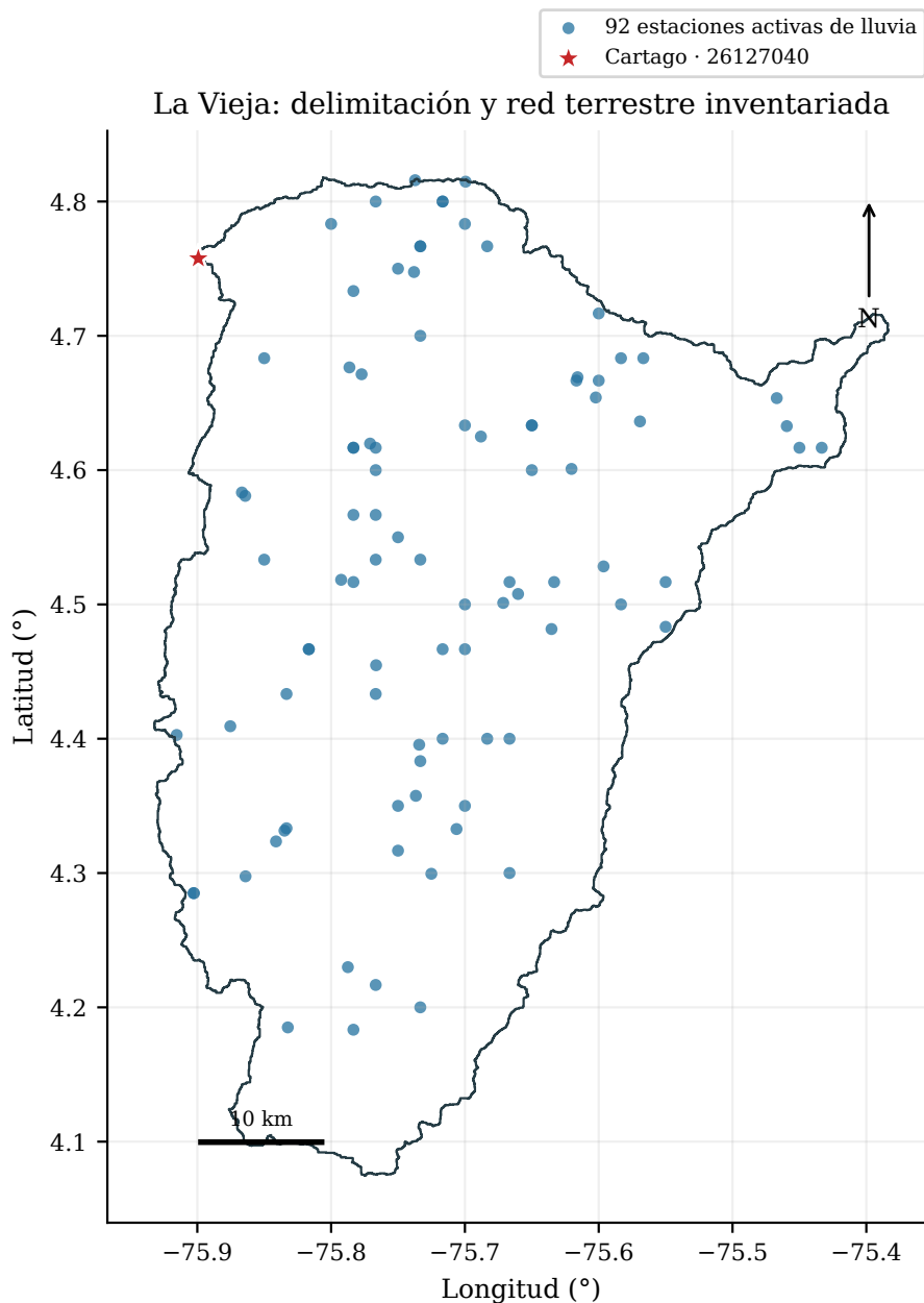
Figura 6: Cuenca La Vieja hasta Cartago y estaciones terrestres inventariadas.
