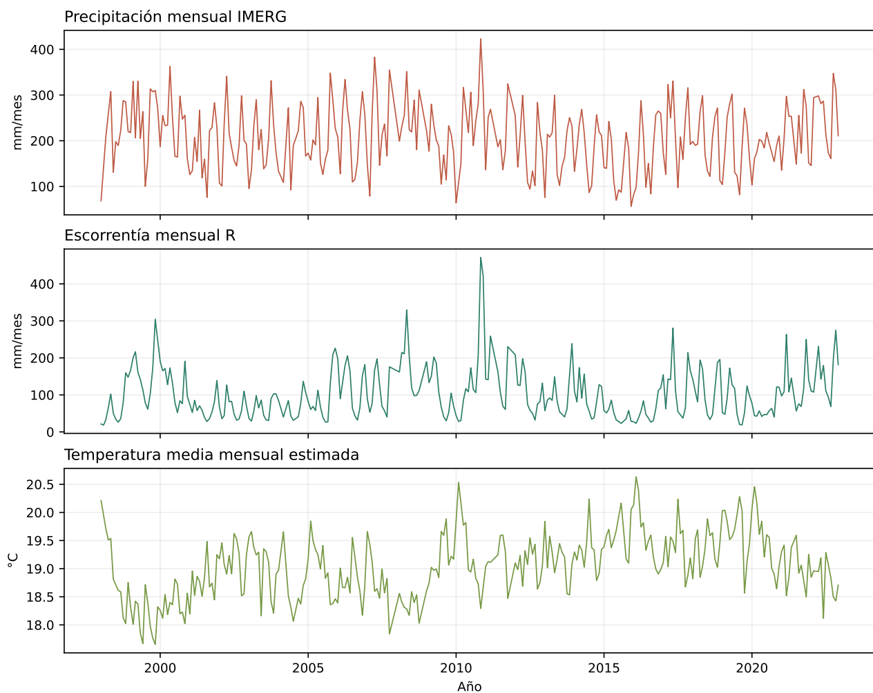
Figura 12: IMERG, escoorrentía mensual R y temperatura media mensual estimada, para los 285 meses completos simultáneos. IMERG y R están en mm/mes.
